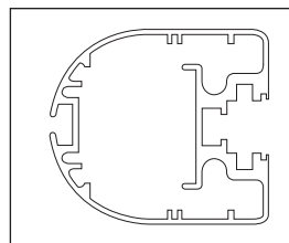
Profil 80x70mm
